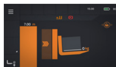
Horquillas inclinadas y desplazadas lateralmente
